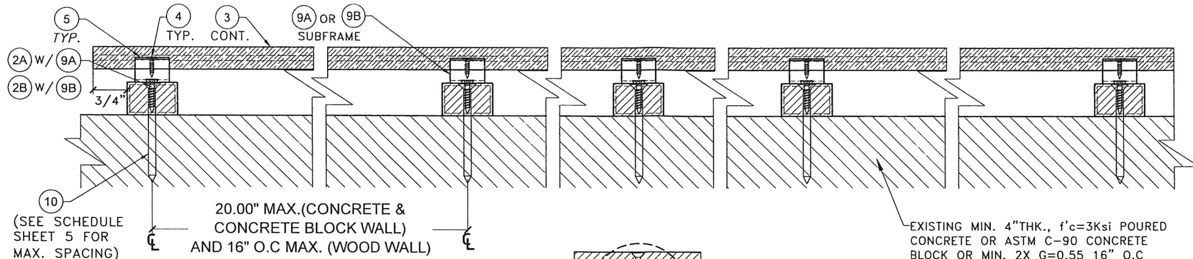
SECTION B-B N.T.S
