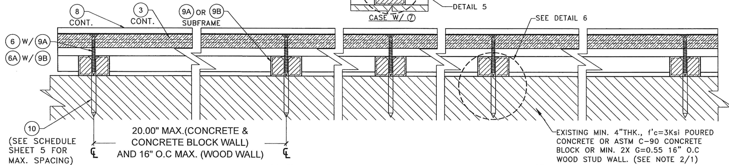
SECTION C-C N.T.S
